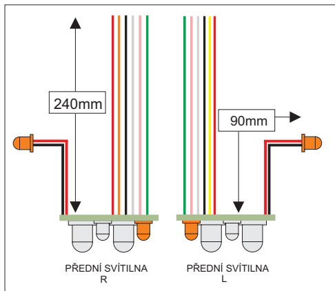
PŘEDNÍ SVĚTLA
