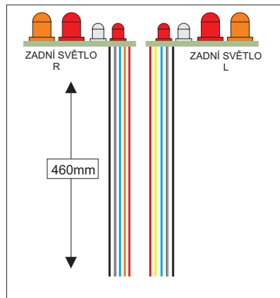
ZADNÍ SVĚTLA
