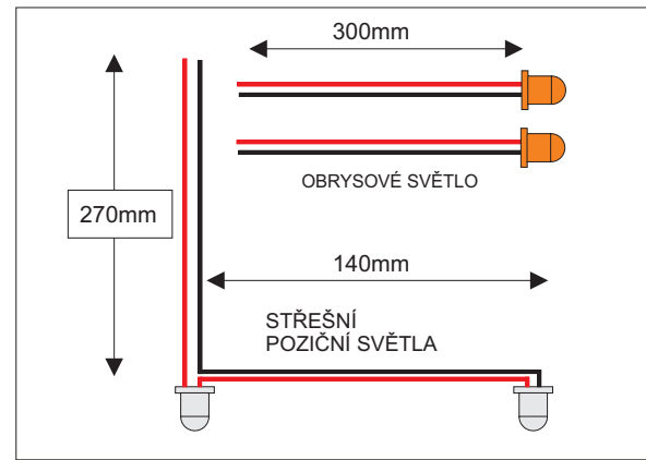
OBRYSOVÁ SVĚTLA
