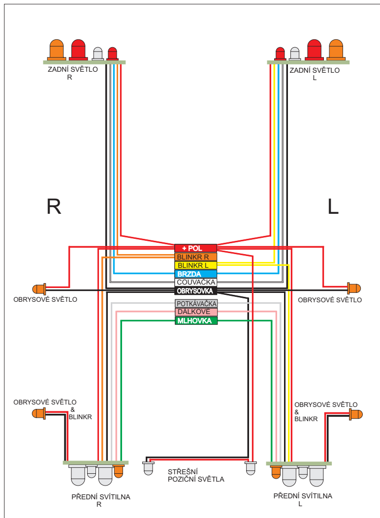
PŘEDNÍ SVĚTLA
